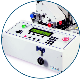
LCD Display
